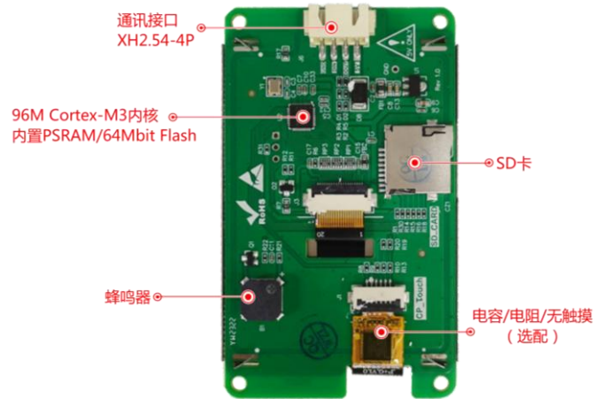
图 1-3 硬件配置图
