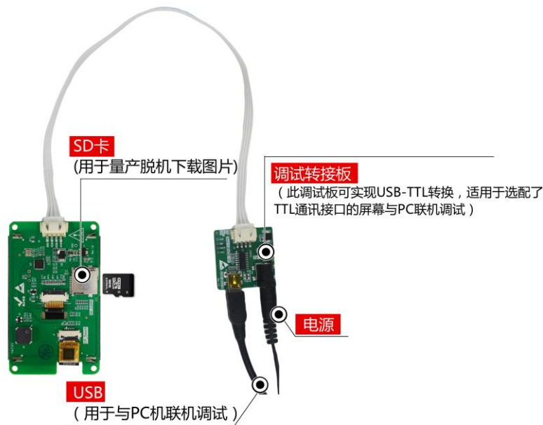
图 1-4 调试工具图
